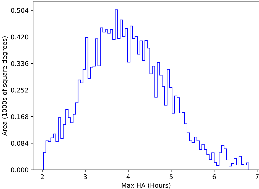
roman_v3.3_10yrs WFD u band: Max HA
