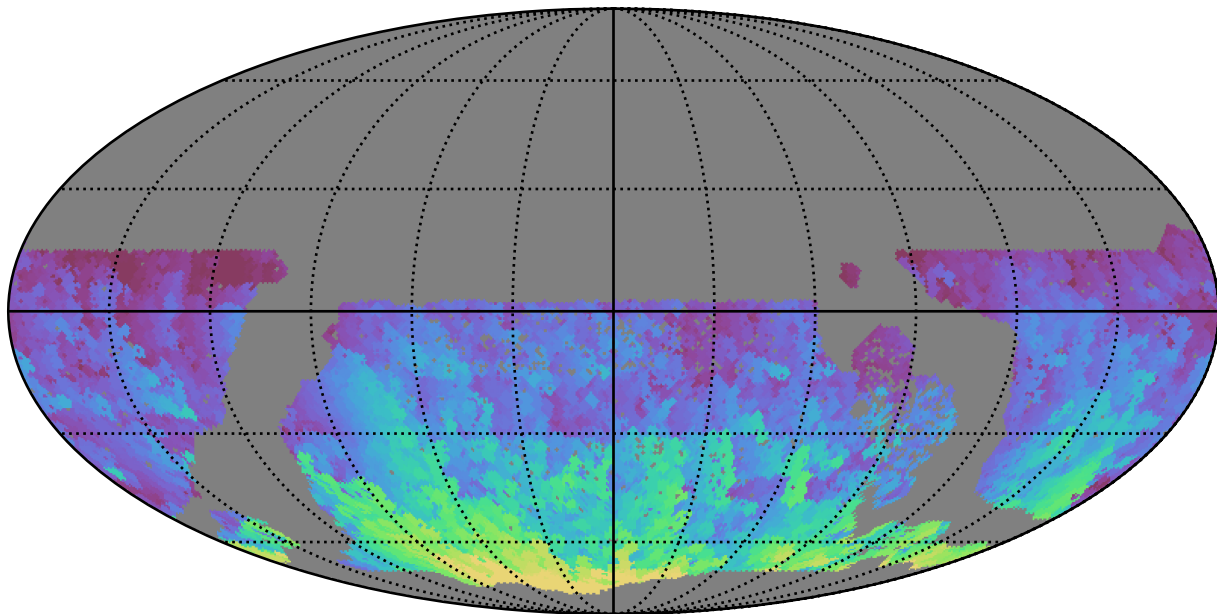
roman_v3.3_10yrs WFD r band: Max HA
