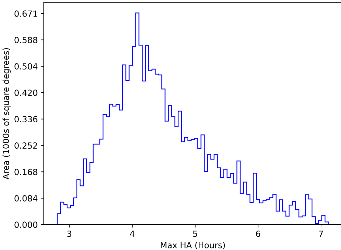
roman_v3.3_10yrs WFD r band: Max HA
