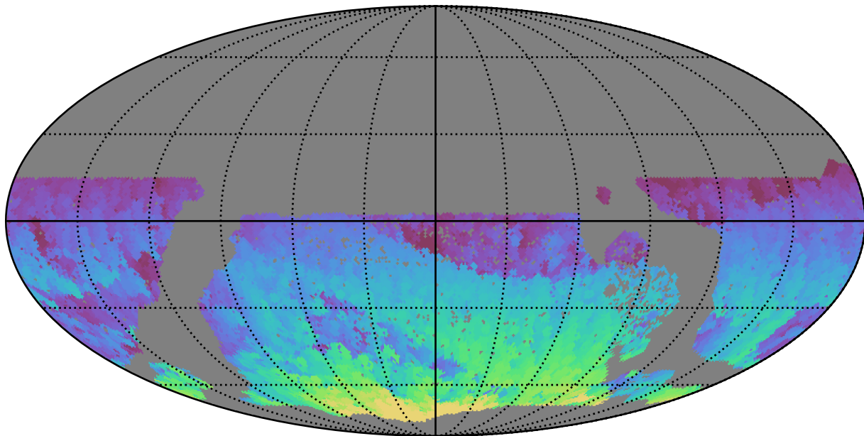
roman_v3.3_10yrs WFD i band: Max HA
