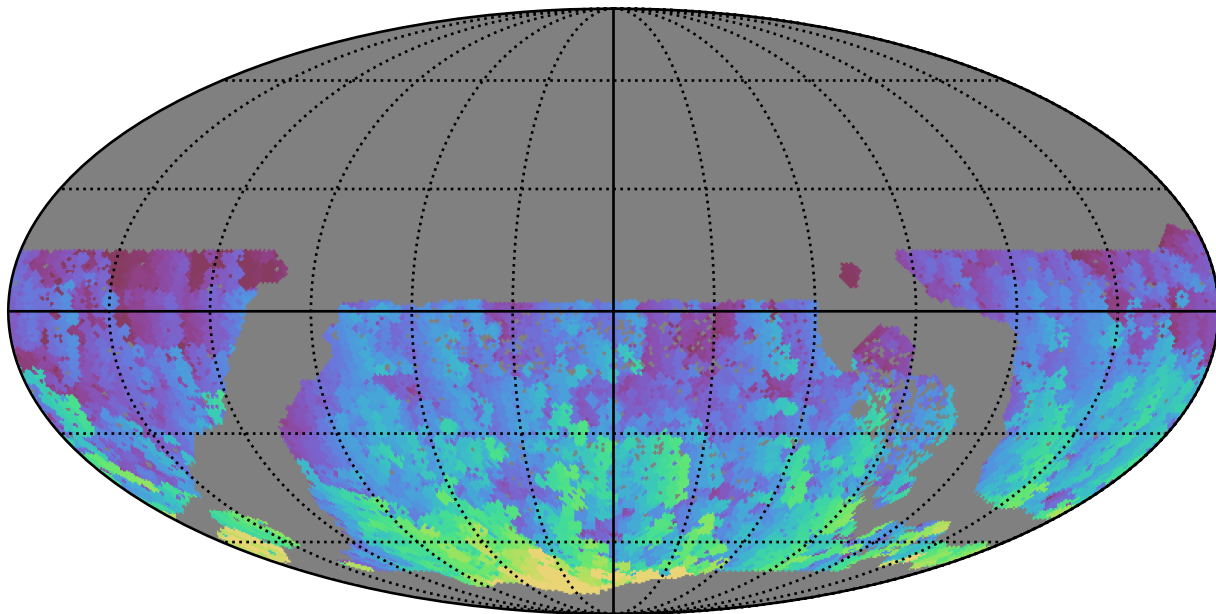
roman_v3.3_10yrs WFD g band: Max HA
