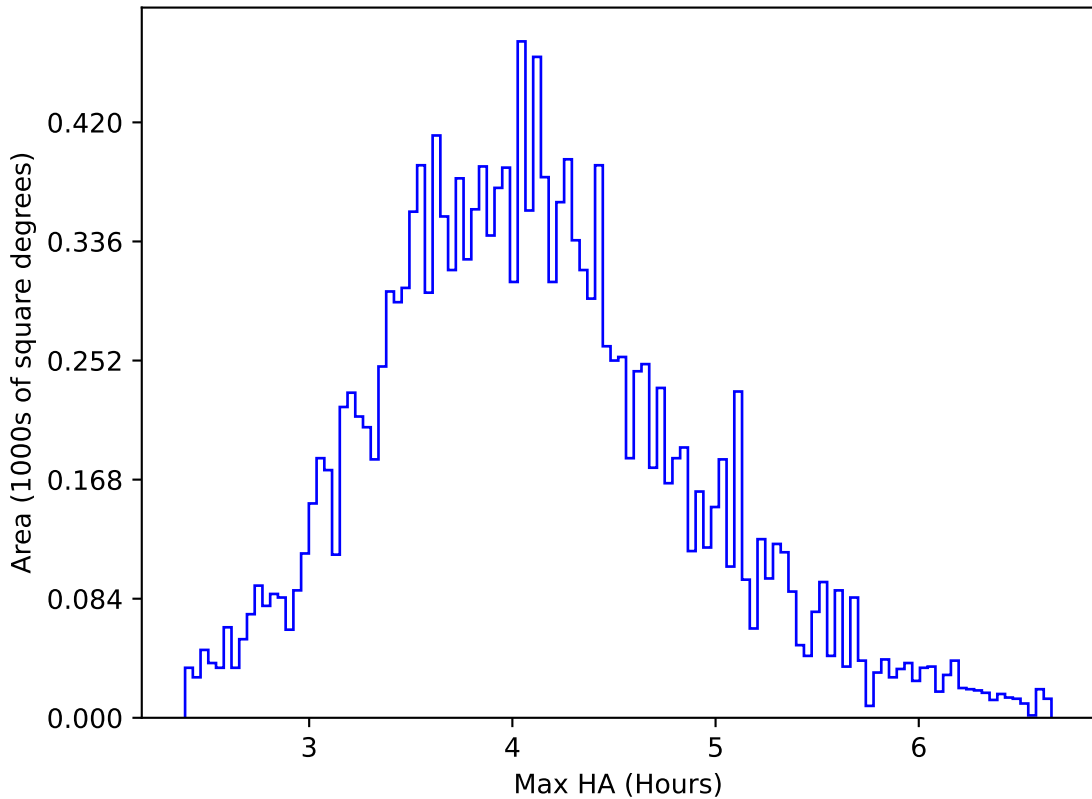
roman_v3.3_10yrs WFD g band: Max HA
