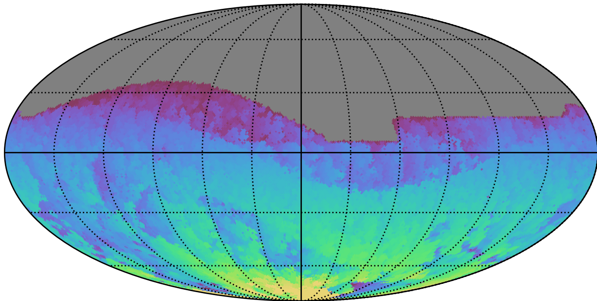
roman_v3.3_10yrs All sky z band: Max HA
