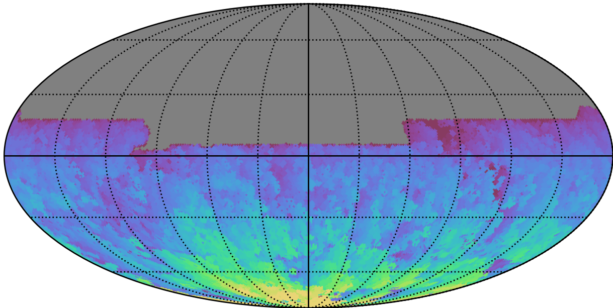
roman_v3.3_10yrs All sky y band: Max HA
