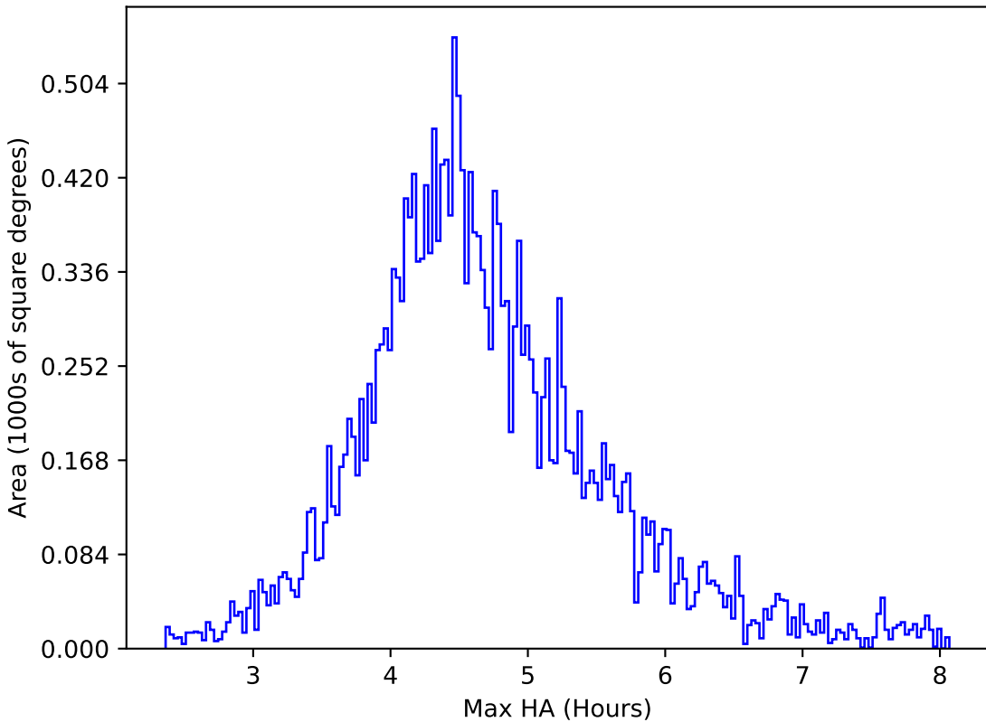
roman_v3.3_10yrs All sky y band: Max HA
