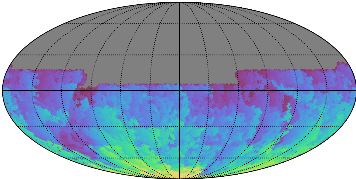
roman_v3.3_10yrs All sky u band: Max HA
