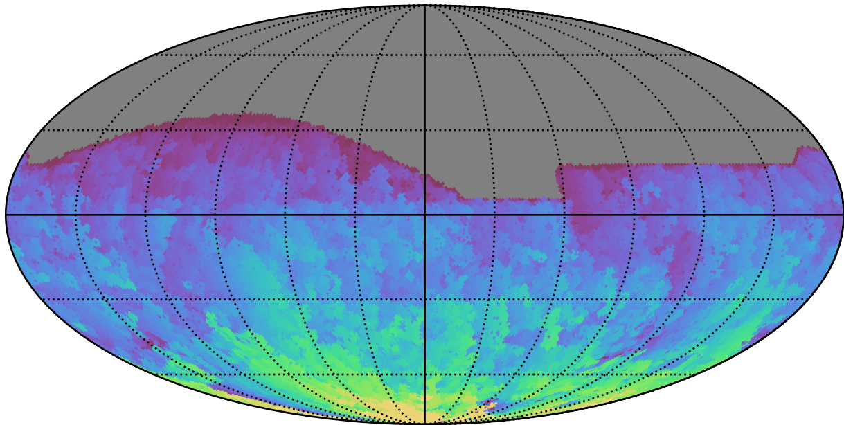
roman_v3.3_10yrs All sky r band: Max HA
