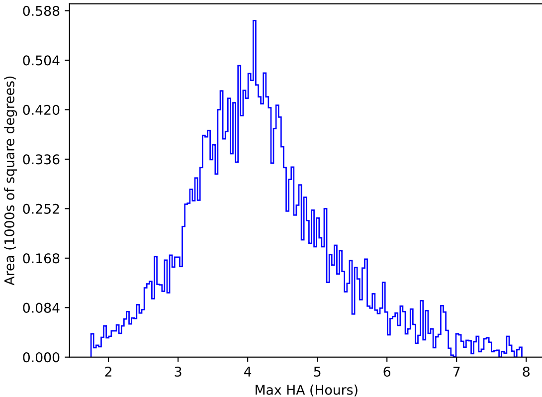
roman_v3.3_10yrs All sky r band: Max HA
