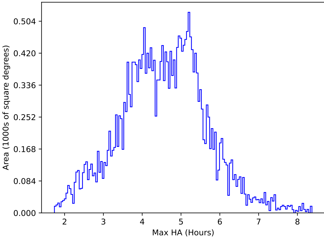
roman_v3.3_10yrs All sky i band: Max HA
