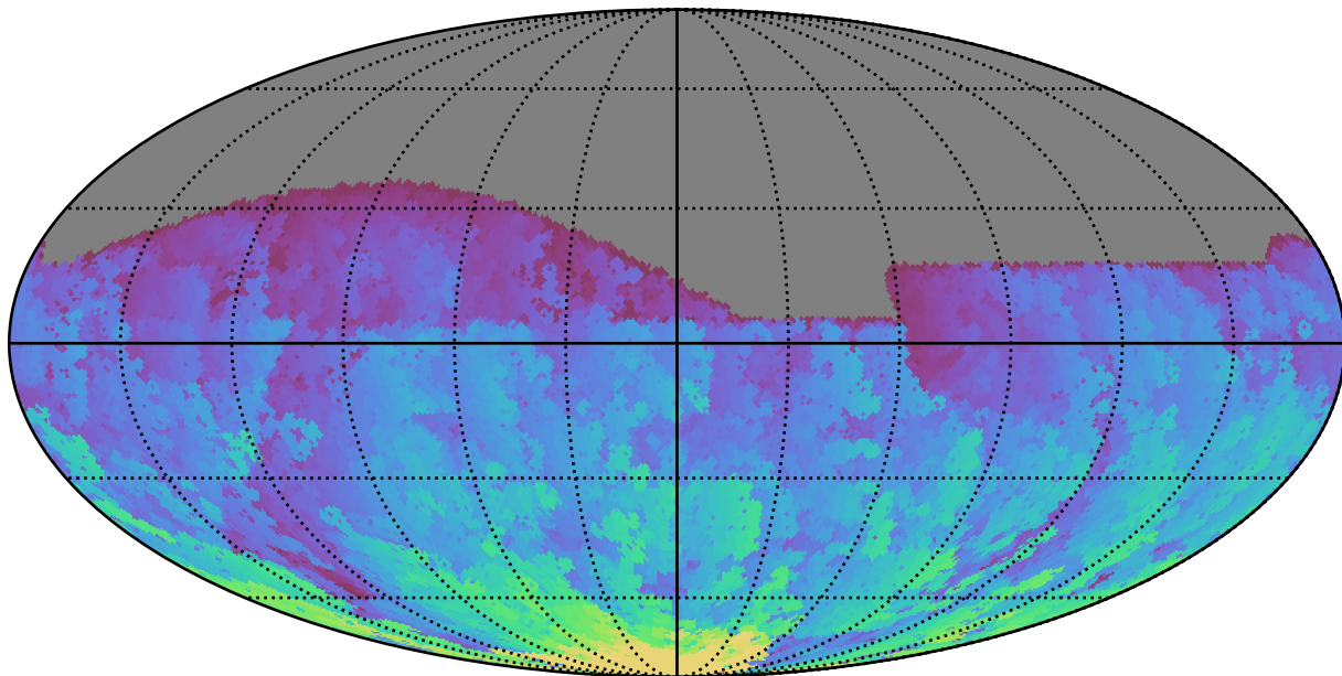
roman_v3.3_10yrs All sky g band: Max HA
