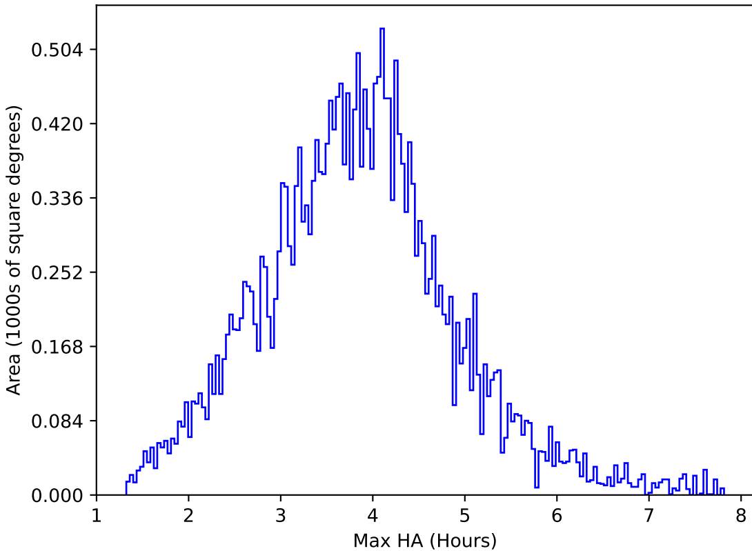
roman_v3.3_10yrs All sky g band: Max HA
