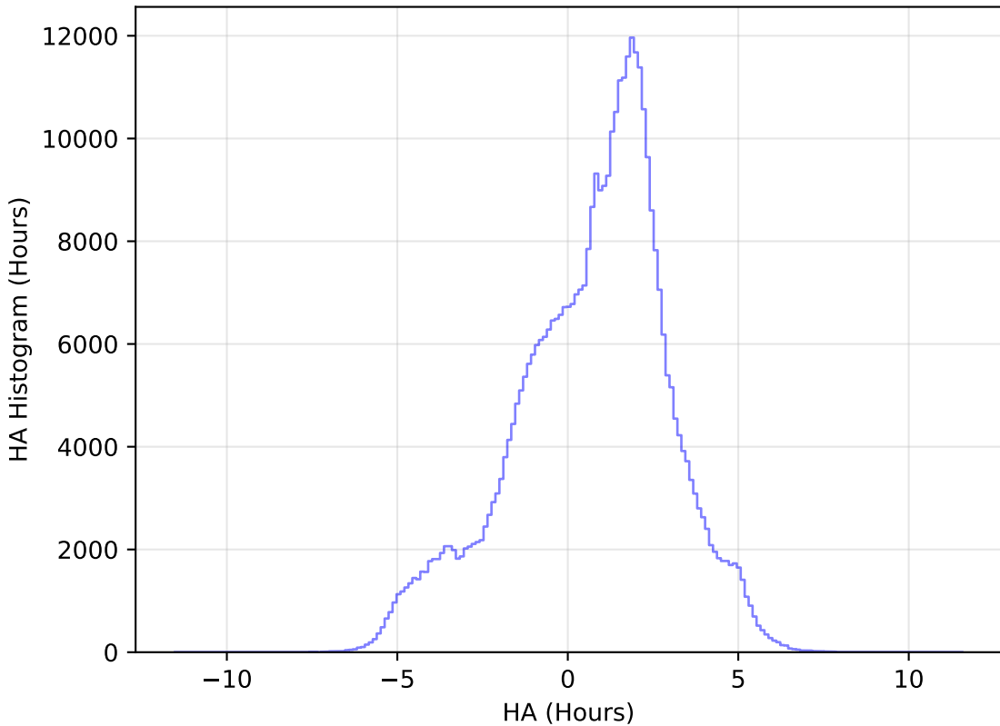
roman_v3.3_10yrs WFD z band: HA Histogram
