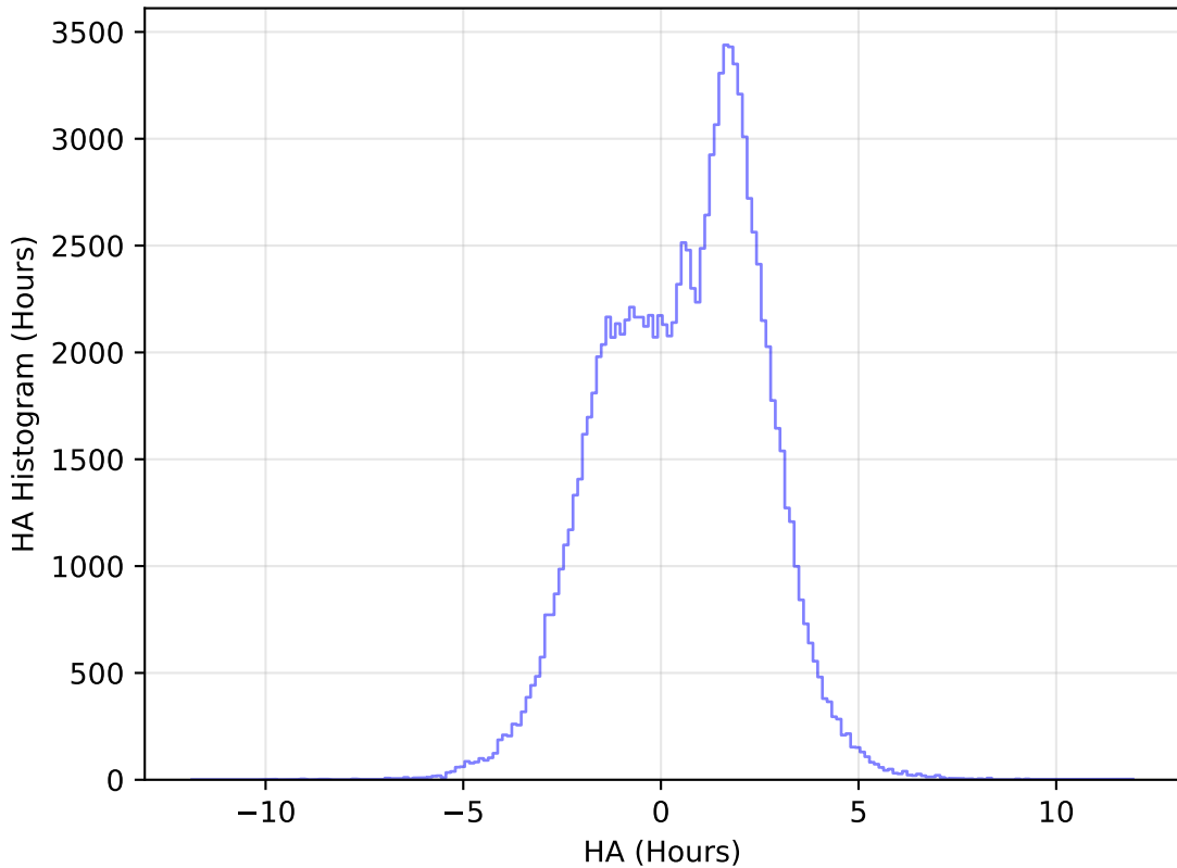
roman_v3.3_10yrs WFD u band: HA Histogram
