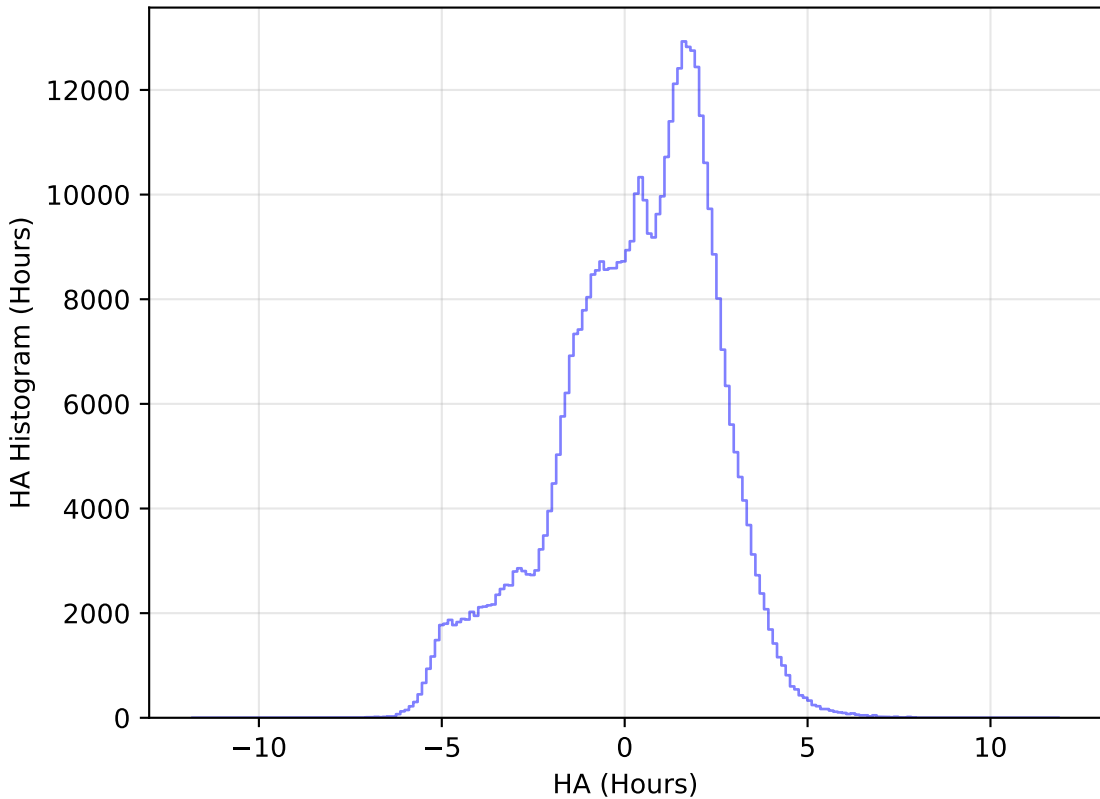
roman_v3.3_10yrs WFD r band: HA Histogram
