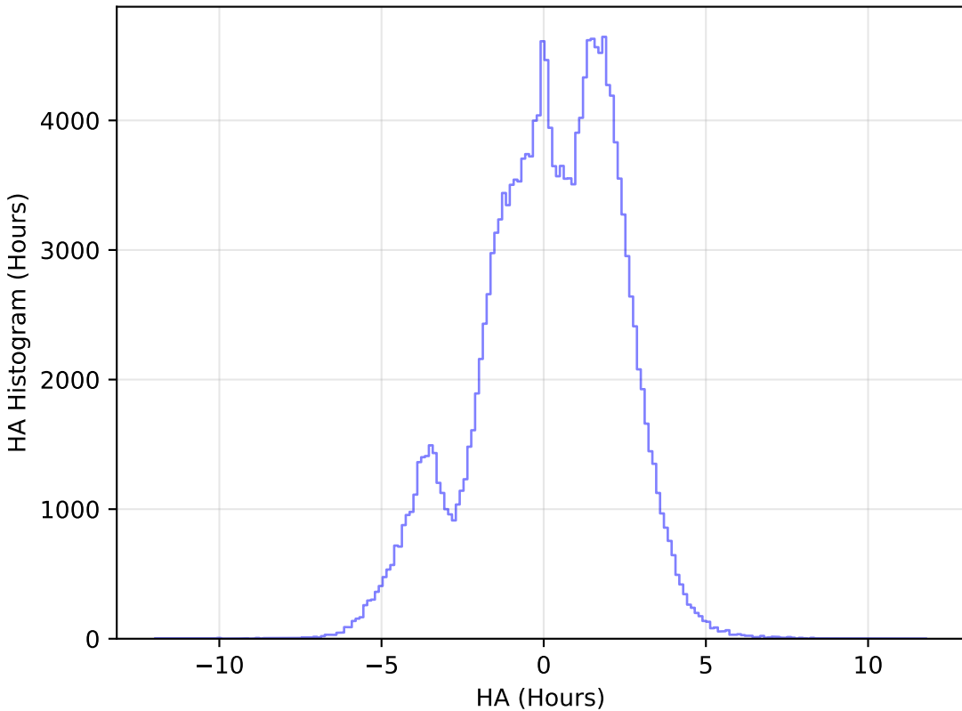
roman_v3.3_10yrs WFD g band: HA Histogram
