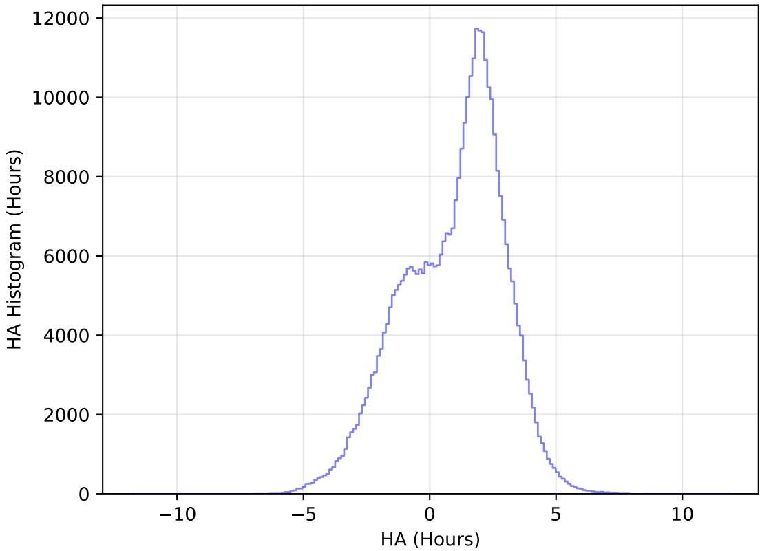
roman_v3.3_10yrs All sky y band: HA Histogram
