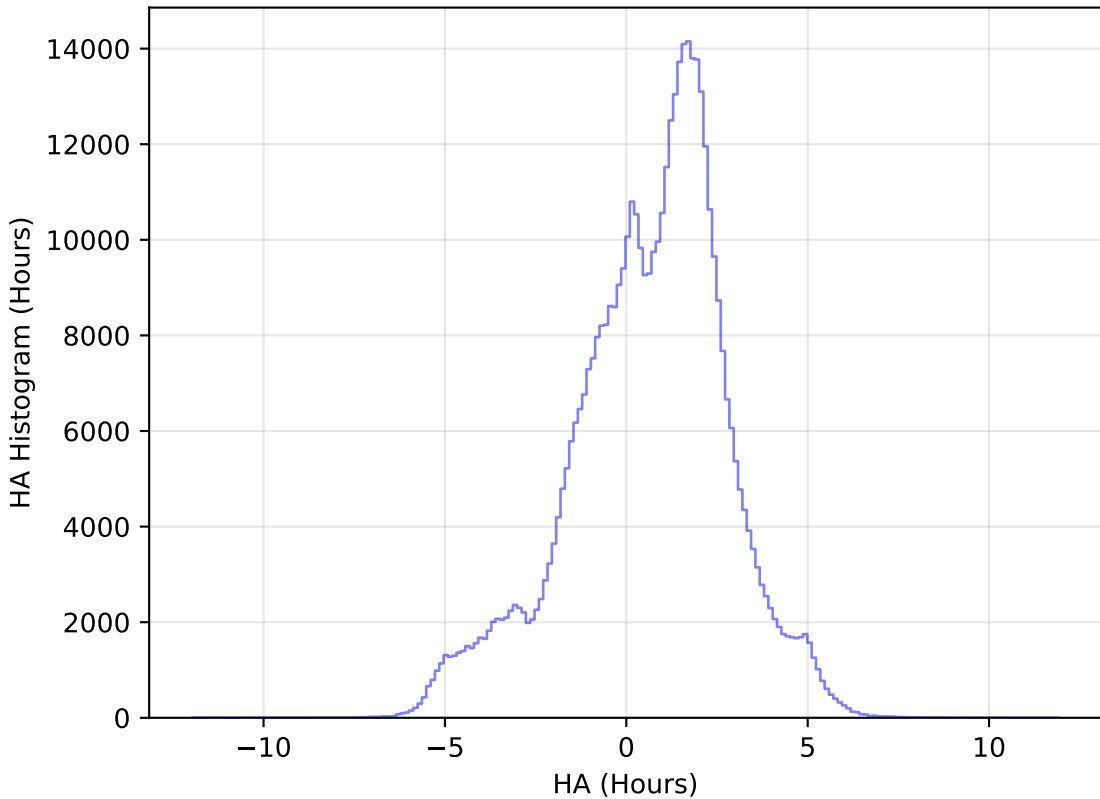
roman_v3.3_10yrs All sky i band: HA Histogram
