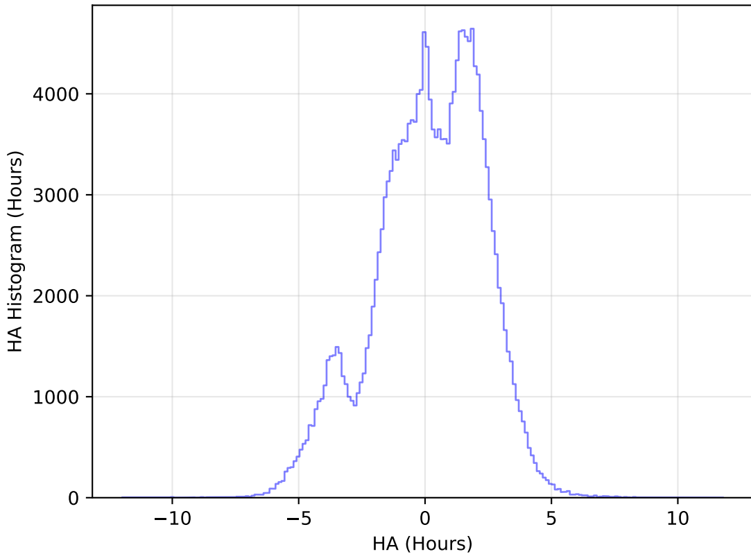
roman_v3.3_10yrs All sky g band: HA Histogram
