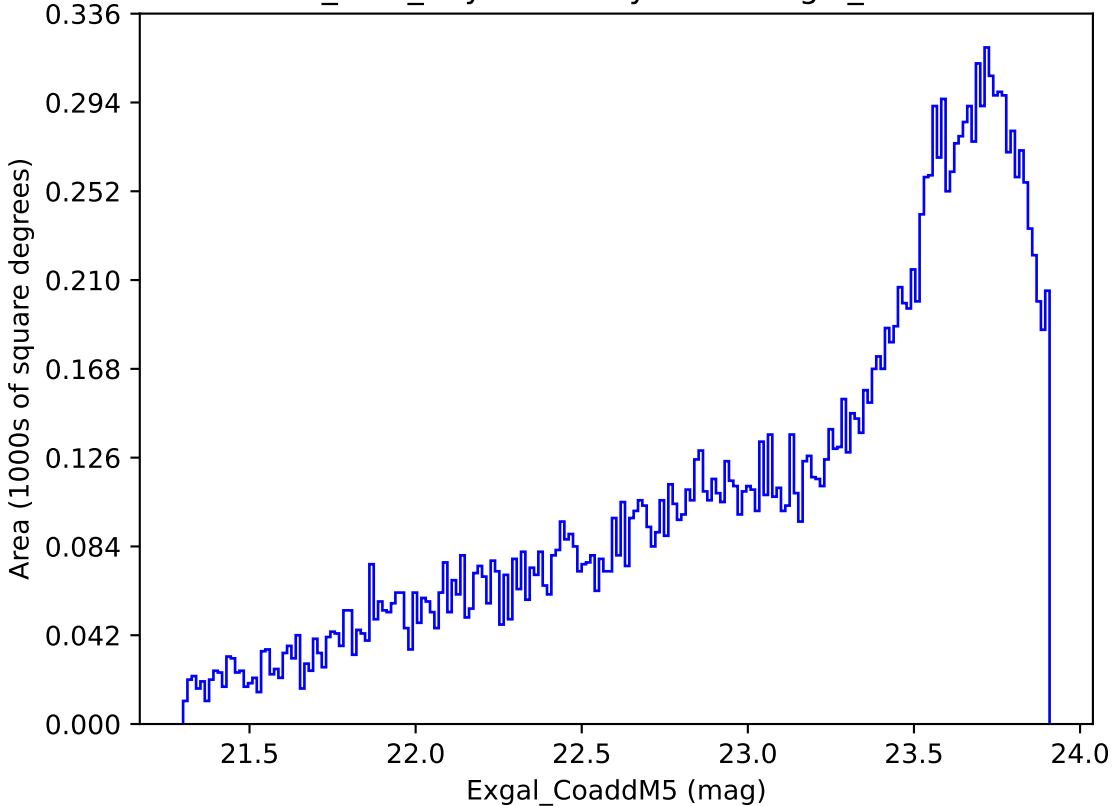
roman_v3.3_10yrs Yr 3-4 y band: Exgal_CoaddM5
