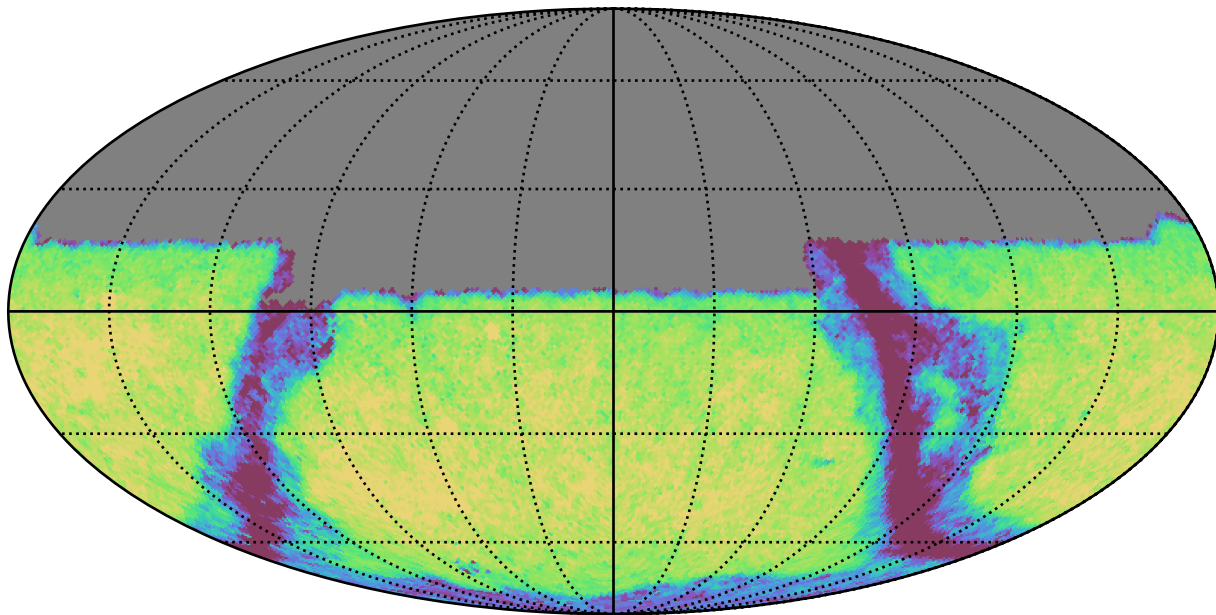
roman_v3.3_10yrs Yr 1 y band: Exgal_CoaddM5
