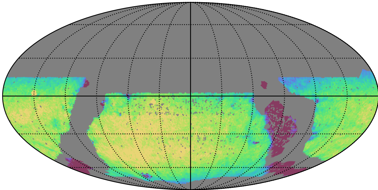
roman_v3.3_10yrs WFD y band: Exgal_CoaddM5
