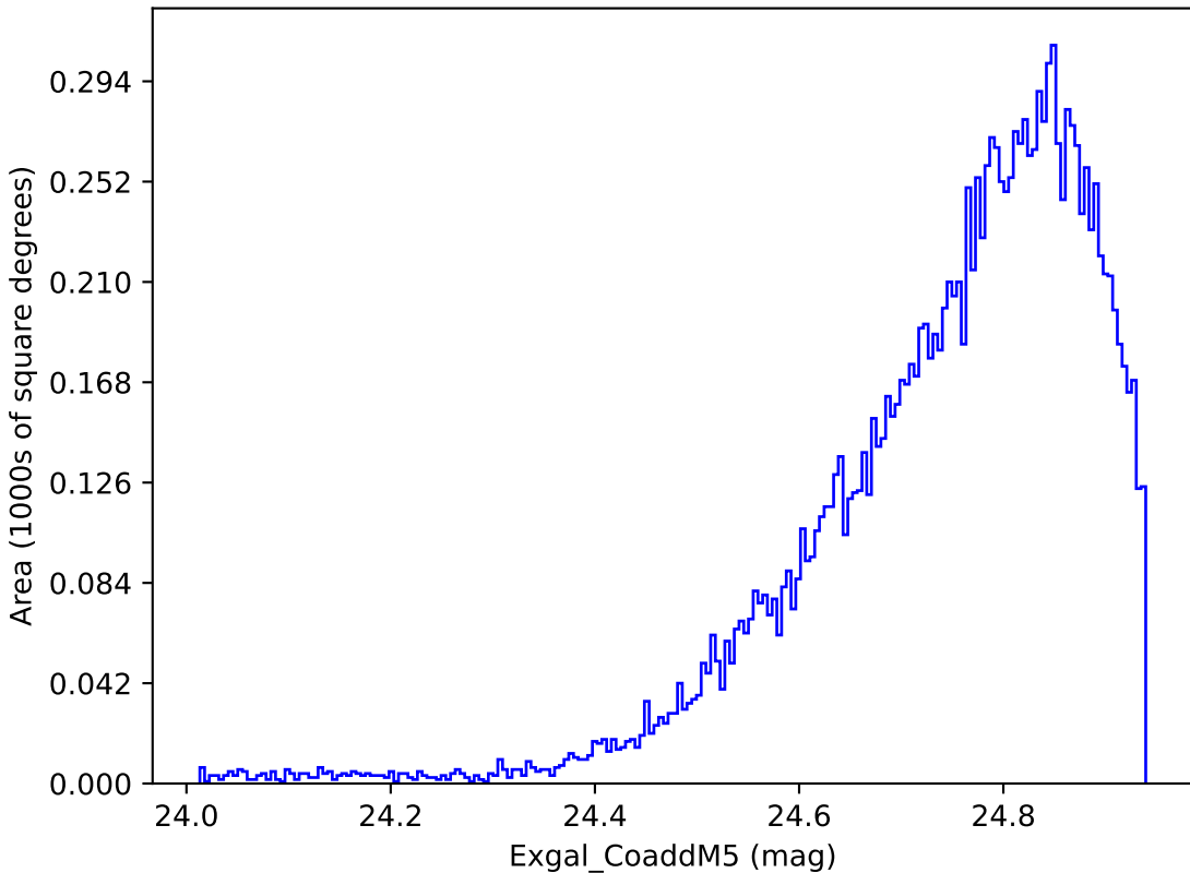
roman_v3.3_10yrs WFD y band: Exgal_CoaddM5
