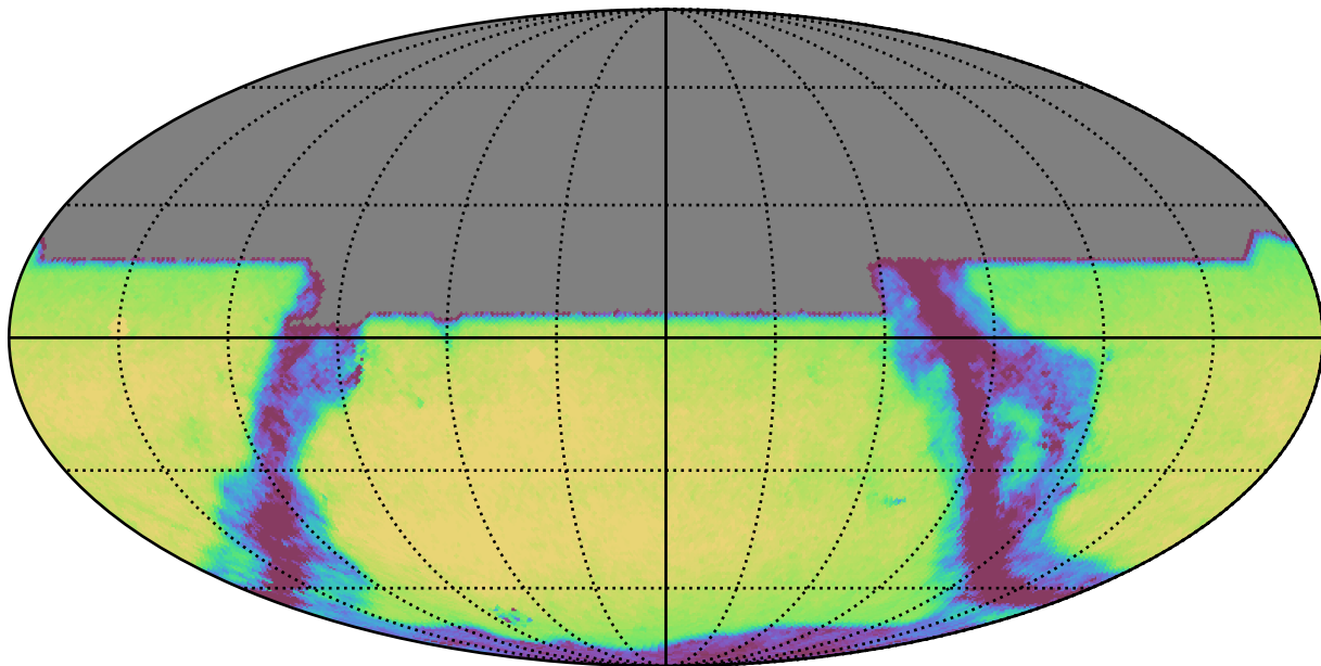
roman_v3.3_10yrs All sky y band: Exgal_CoaddM5
