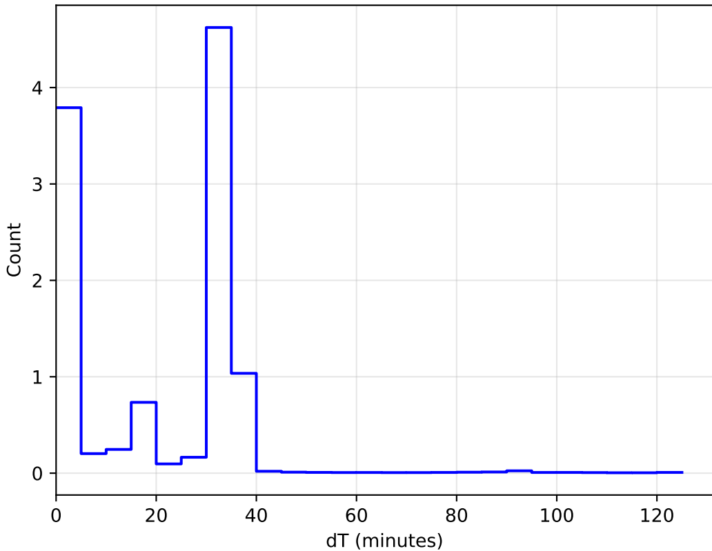
1e6 roman_v3.3_10yrs WFD: DeltaT Histogram
