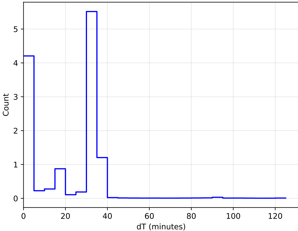
1e6 roman_v3.3_10yrs All sky: DeltaT Histogram
