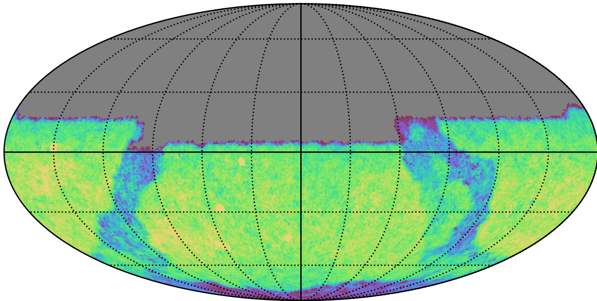
roman_v3.3_10yrs Yr 1 y band: CoaddM5
