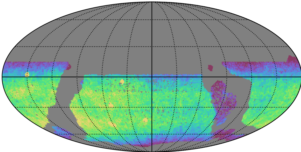
roman_v3.3_10yrs WFD y band: CoaddM5
