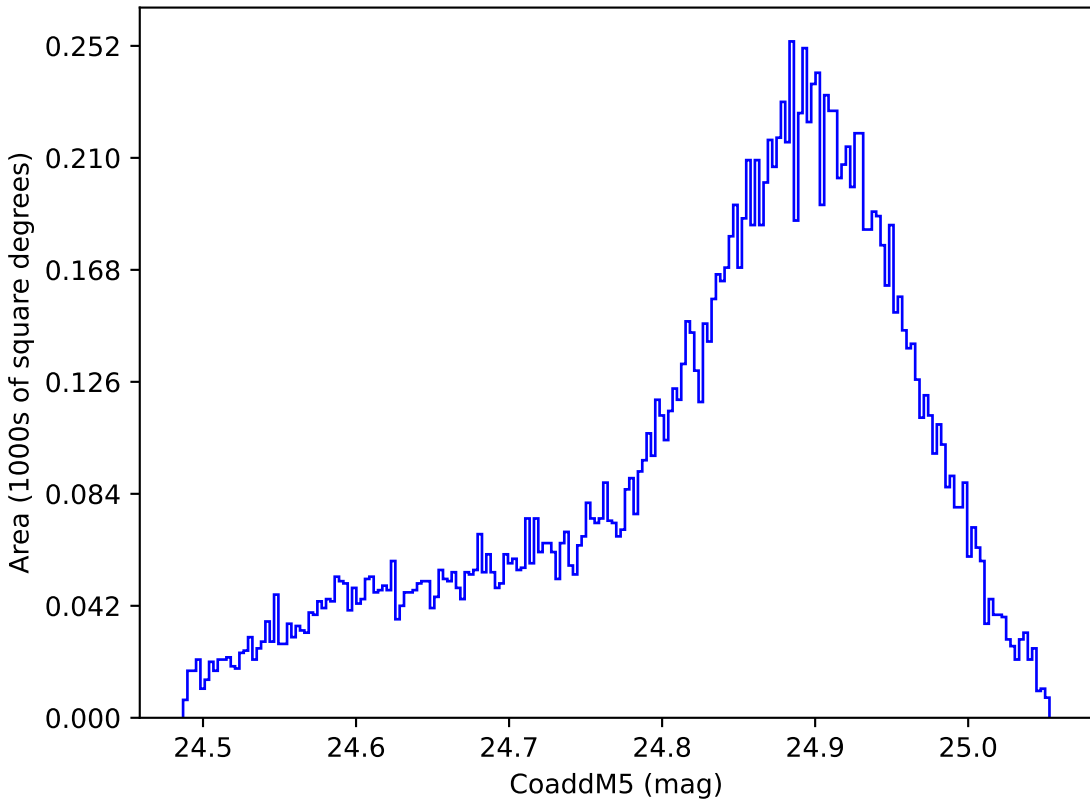
roman_v3.3_10yrs WFD y band: CoaddM5
