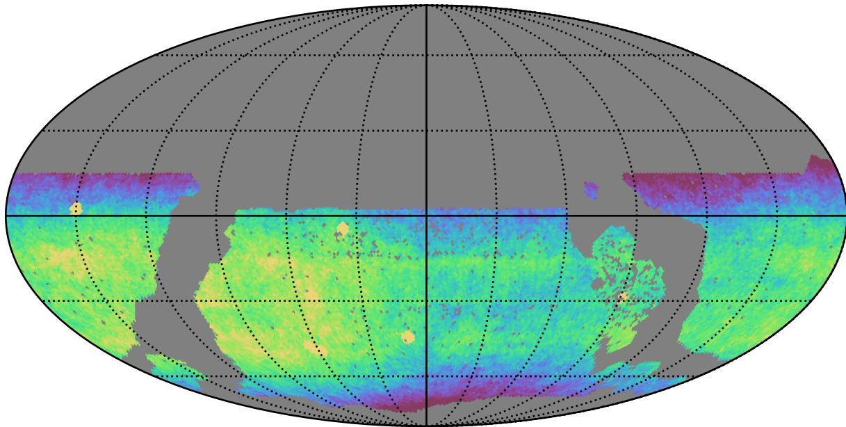
roman_v3.3_10yrs WFD i band: CoaddM5
