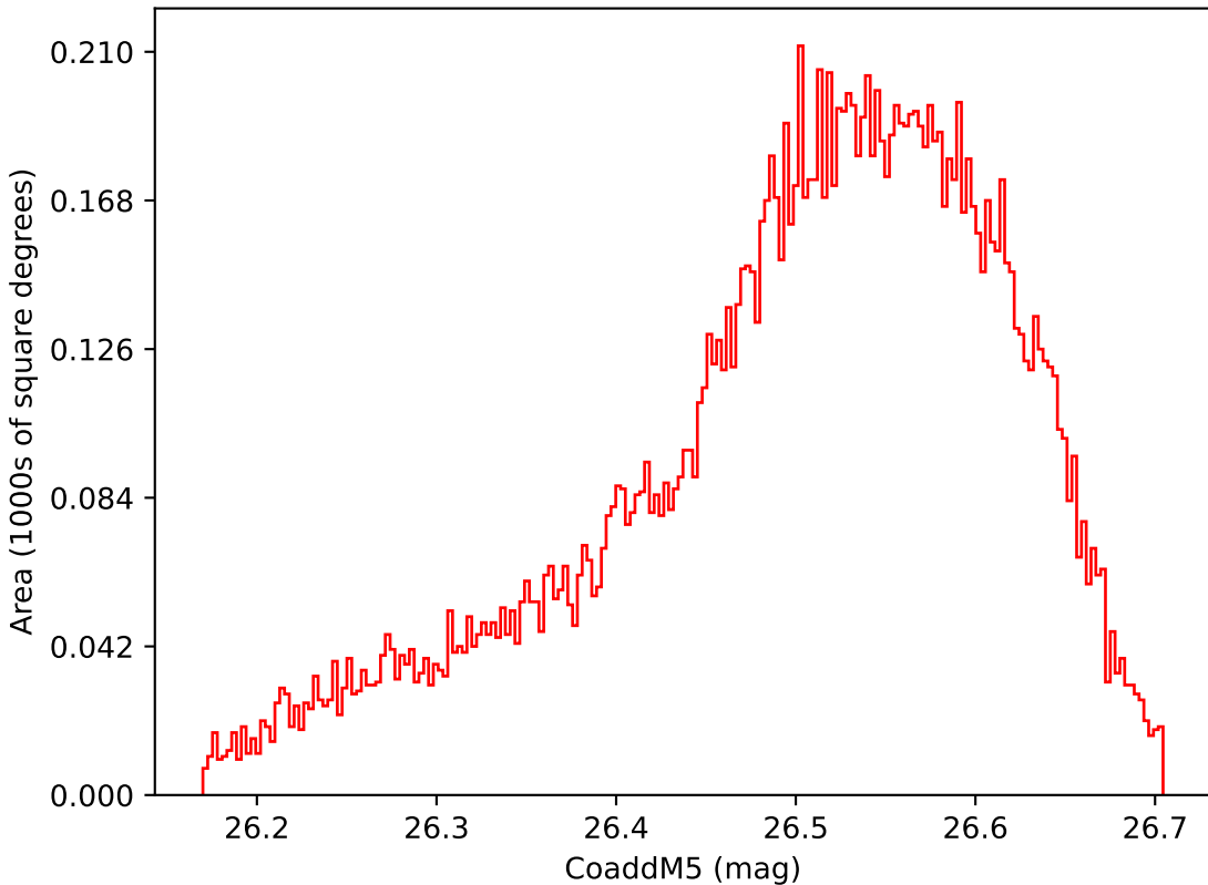
roman_v3.3_10yrs WFD i band: CoaddM5
