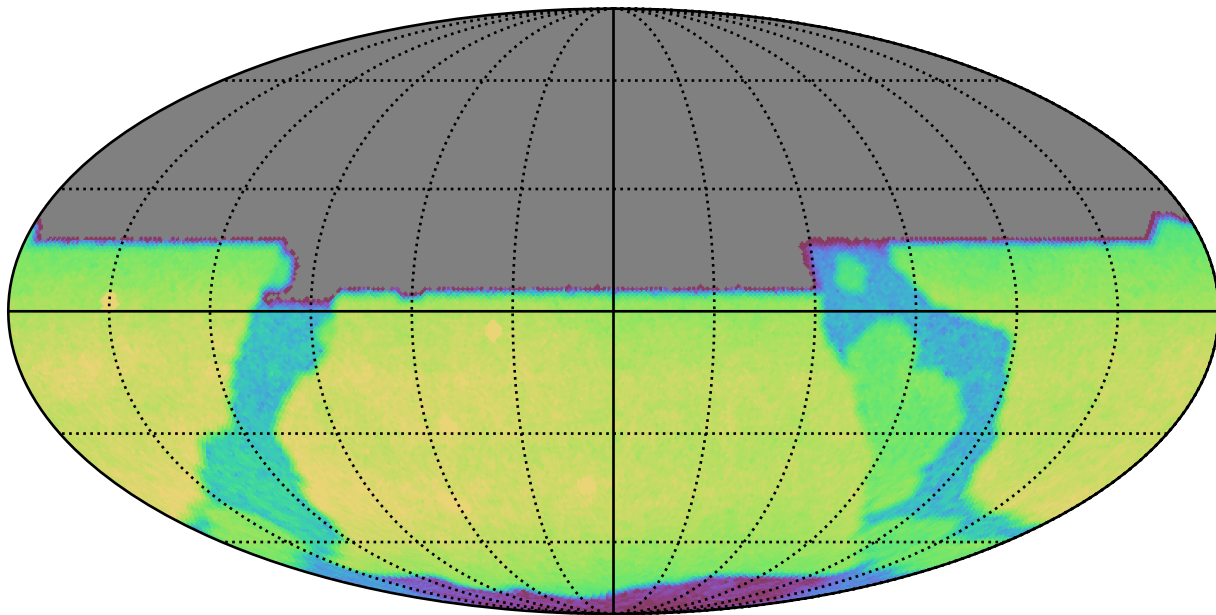
roman_v3.3_10yrs All sky y band: CoaddM5
