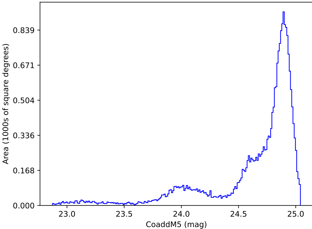
roman_v3.3_10yrs All sky y band: CoaddM5
