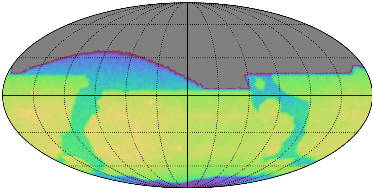
roman_v3.3_10yrs All sky i band: CoaddM5
