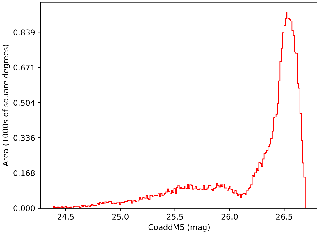
roman_v3.3_10yrs All sky i band: CoaddM5
