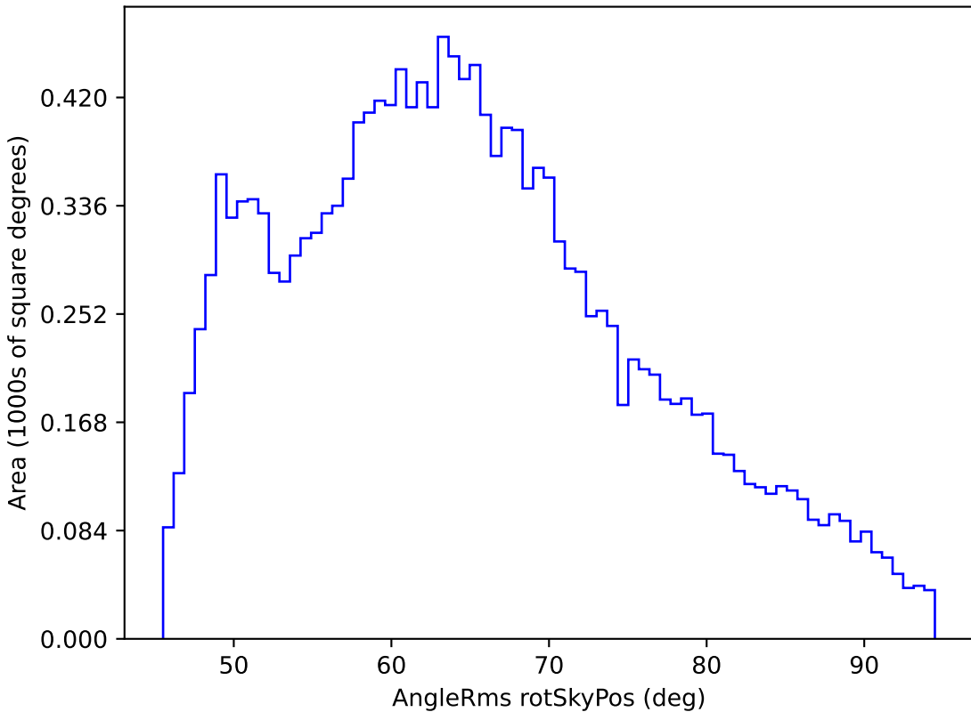
roman_v3.3_10yrs WFD y band: AngleRms rotSkyPos
