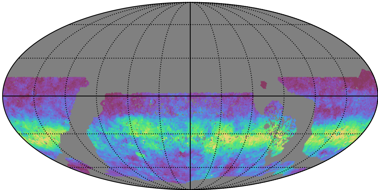
roman_v3.3_10yrs WFD u band: AngleRms rotSkyPos
