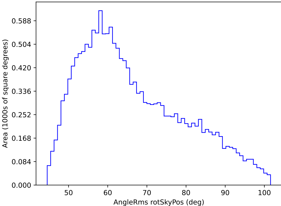
roman_v3.3_10yrs WFD u band: AngleRms rotSkyPos
