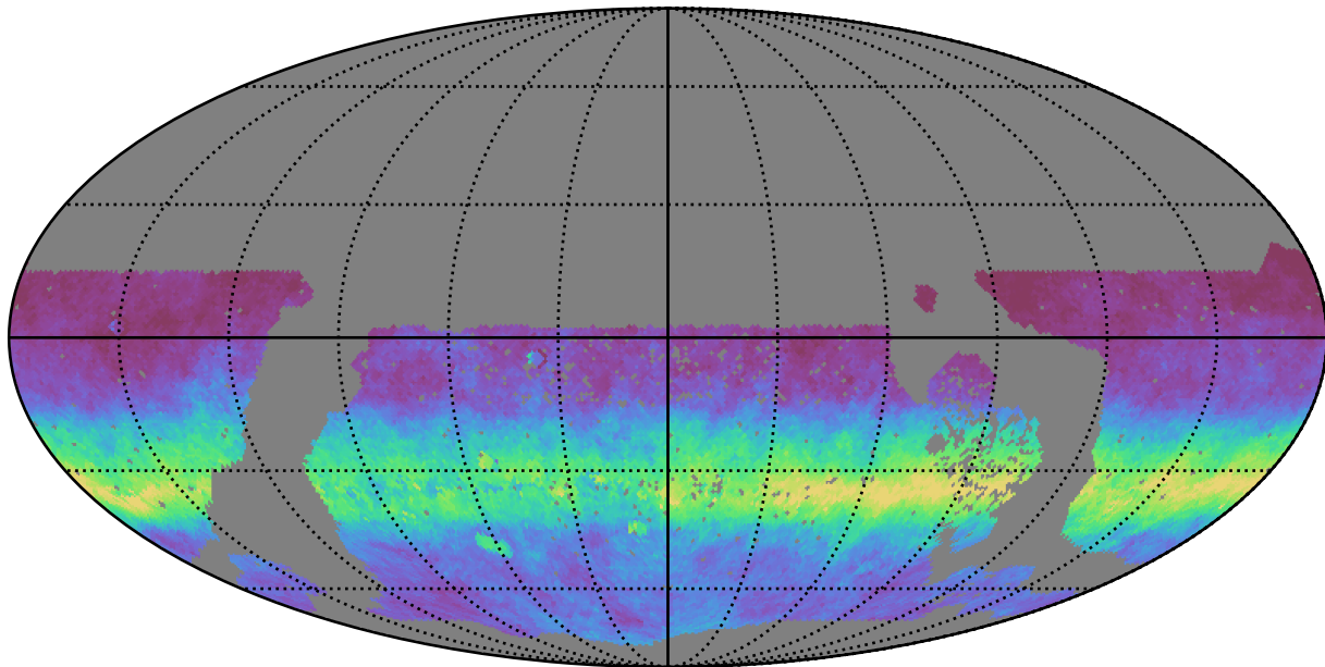
roman_v3.3_10yrs WFD r band: AngleRms rotSkyPos
