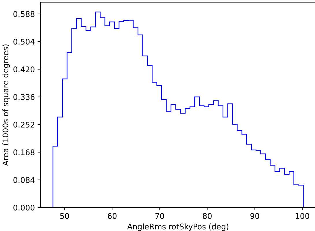
roman_v3.3_10yrs WFD r band: AngleRms rotSkyPos
