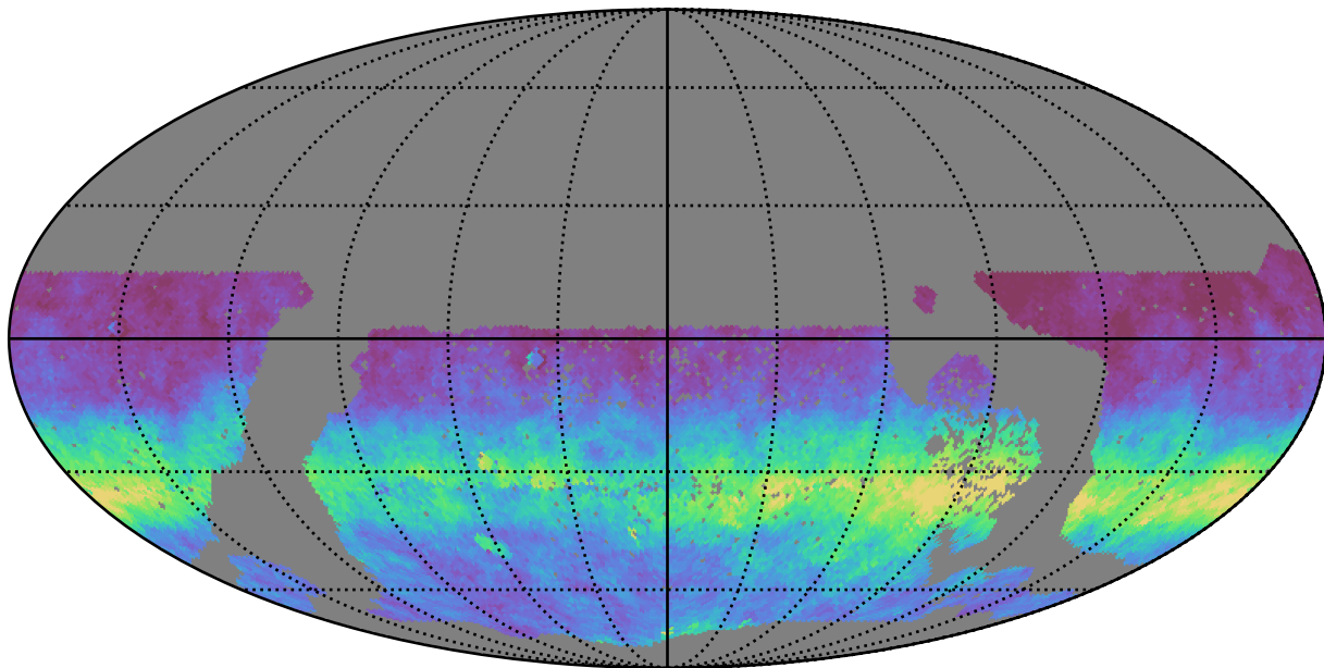
roman_v3.3_10yrs WFD i band: AngleRms rotSkyPos
