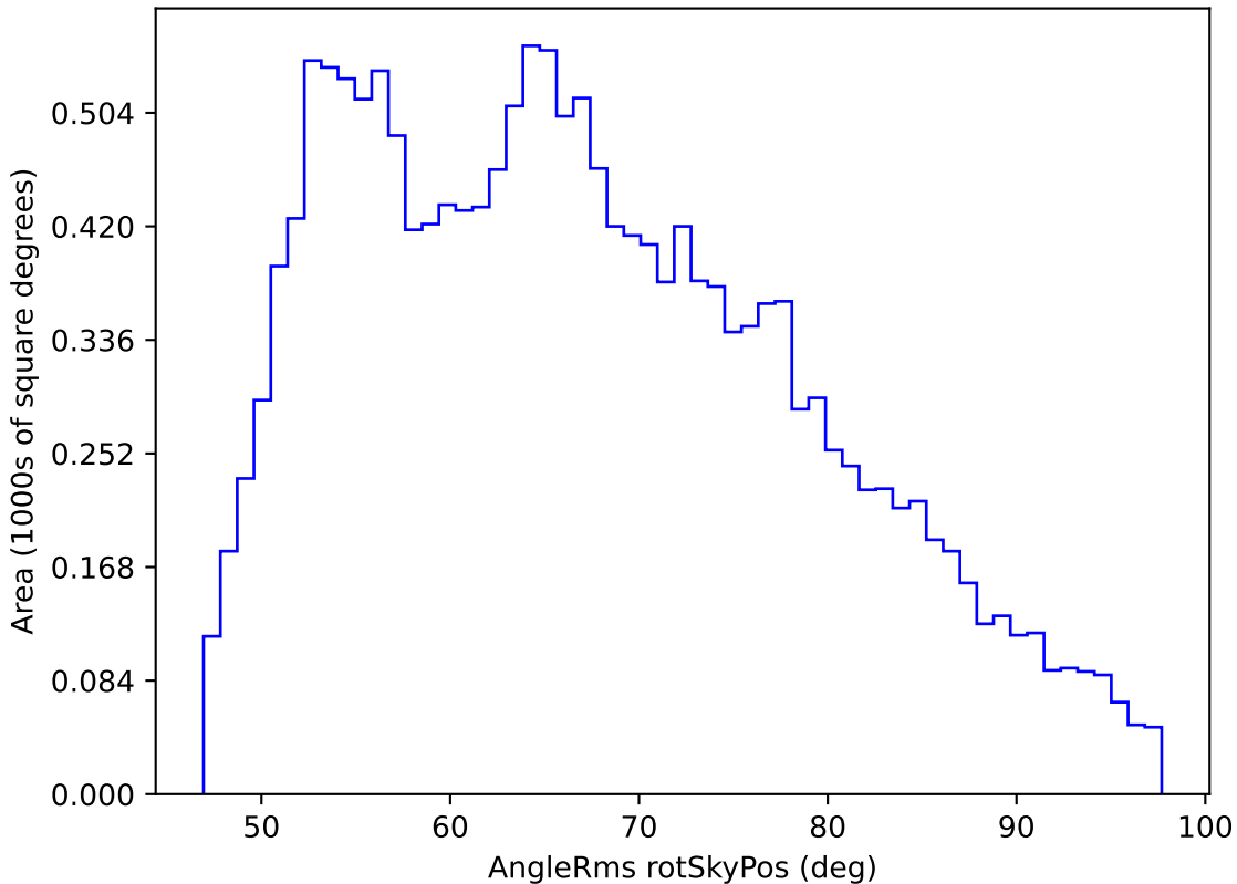
roman_v3.3_10yrs WFD i band: AngleRms rotSkyPos
