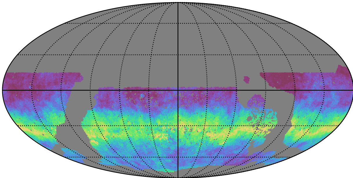
roman_v3.3_10yrs WFD g band: AngleRms rotSkyPos
