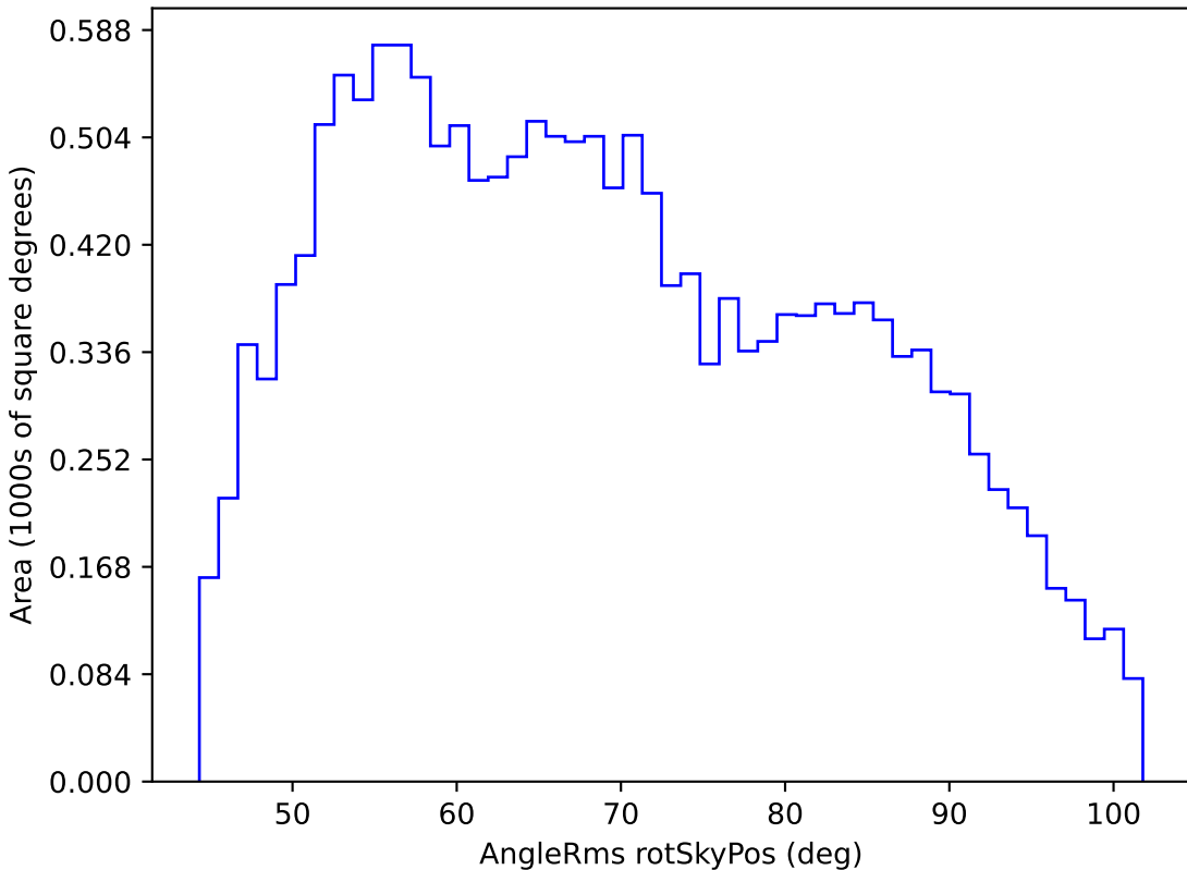
roman_v3.3_10yrs WFD g band: AngleRms rotSkyPos
