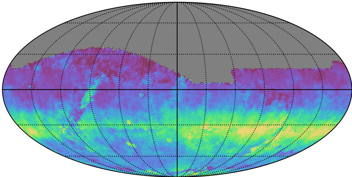
roman_v3.3_10yrs All sky z band: AngleRms rotSkyPos
