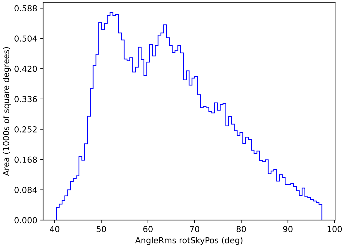
roman_v3.3_10yrs All sky z band: AngleRms rotSkyPos
