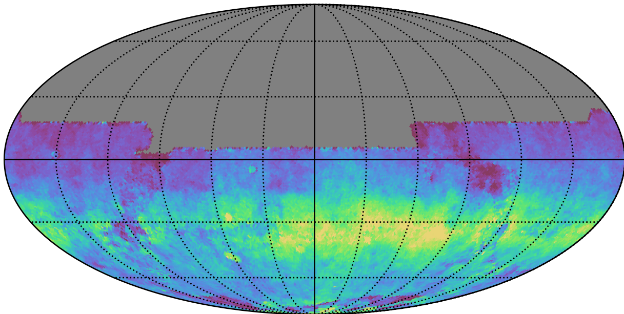
roman_v3.3_10yrs All sky y band: AngleRms rotSkyPos
